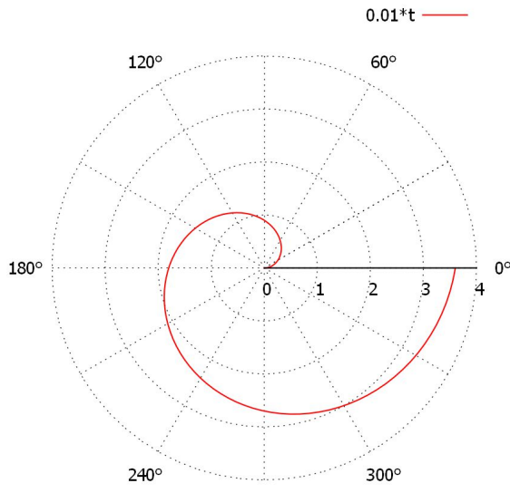
Abbildung 5: Graphische Darstellung einer Funktionen in Polarkoordinaten
